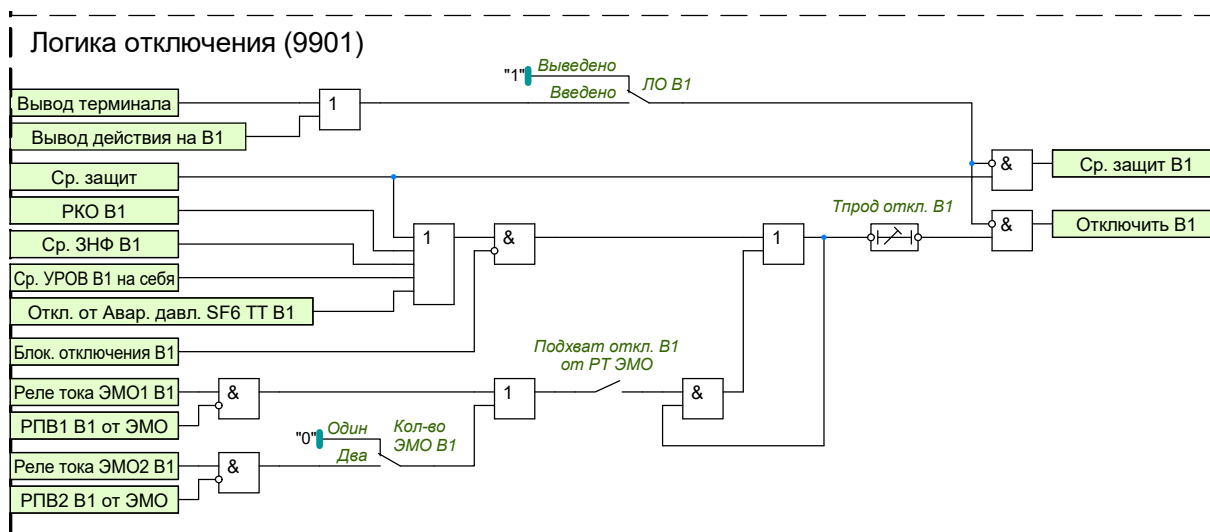
Рисунок 1.52 – Функциональная схема логики отключения В1
