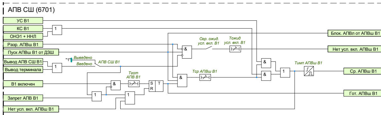
Рисунок 1.41 – Функциональная схема АПВ В1 СШ
