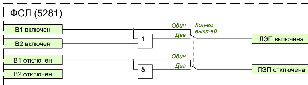
Рисунок 1.55 – Функциональная схема логики ФСЛ
