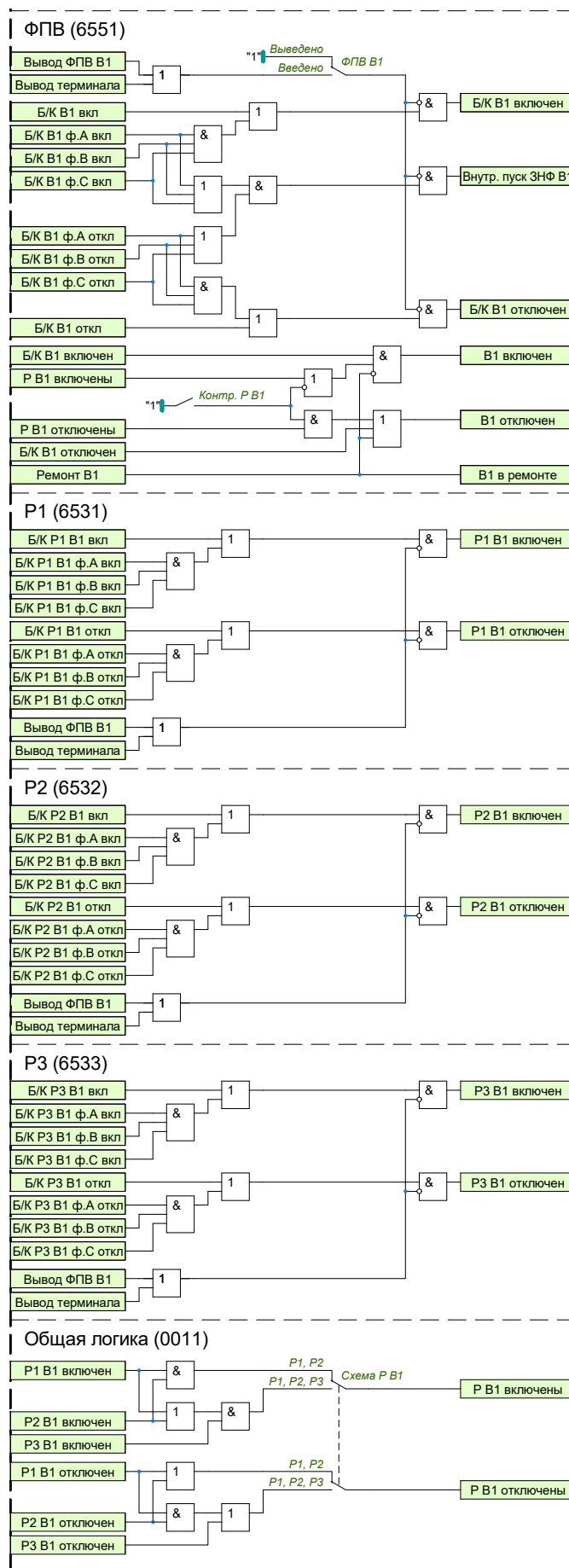
Рисунок 1.54 – Функциональная схема логики ФПВ В1
