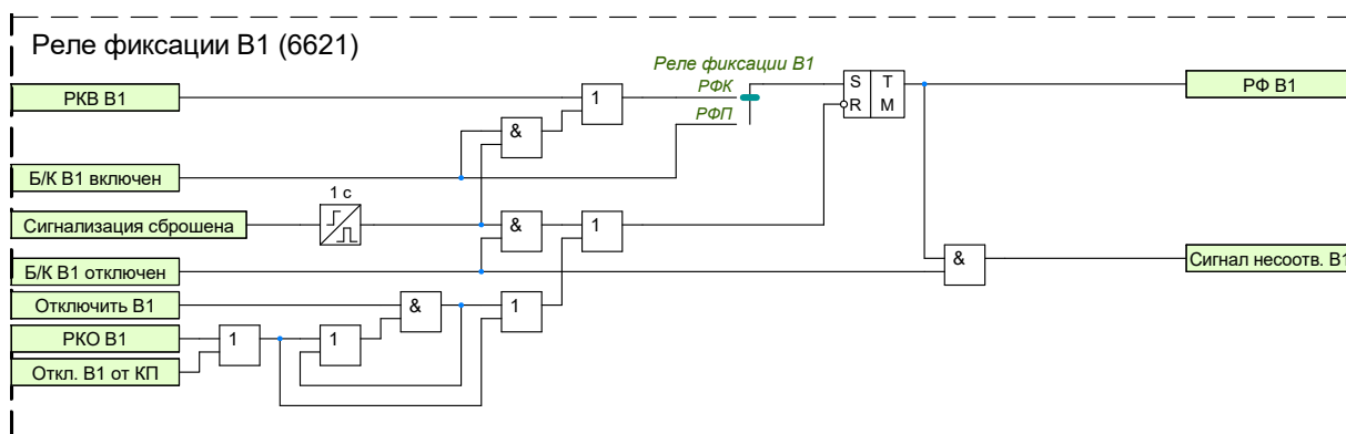
Рисунок 1.50 – Функциональная схема логики реле фиксации В1
