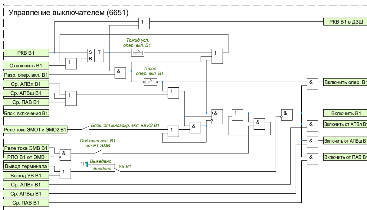
Рисунок 1.53 – Функциональная схема управления выключателем В1
