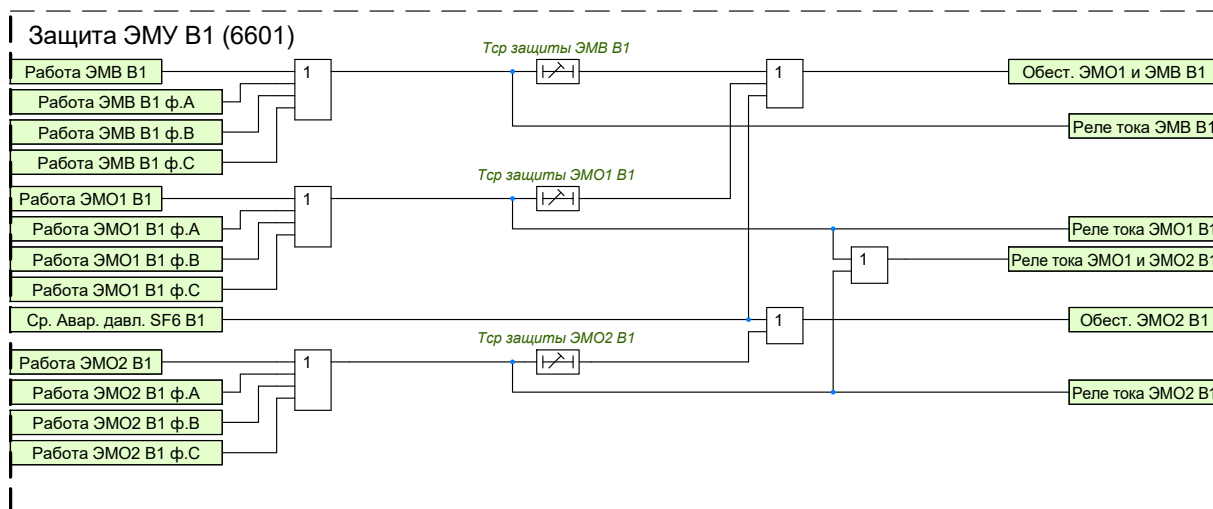
Рисунок 1.48 – Функциональная схема защиты ЭМУ В1
