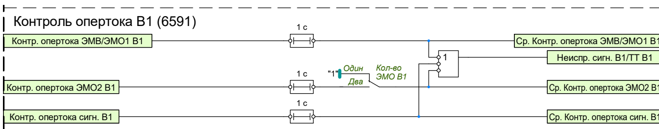
Рисунок 1.47 – Функциональная схема контроля опертока В1
