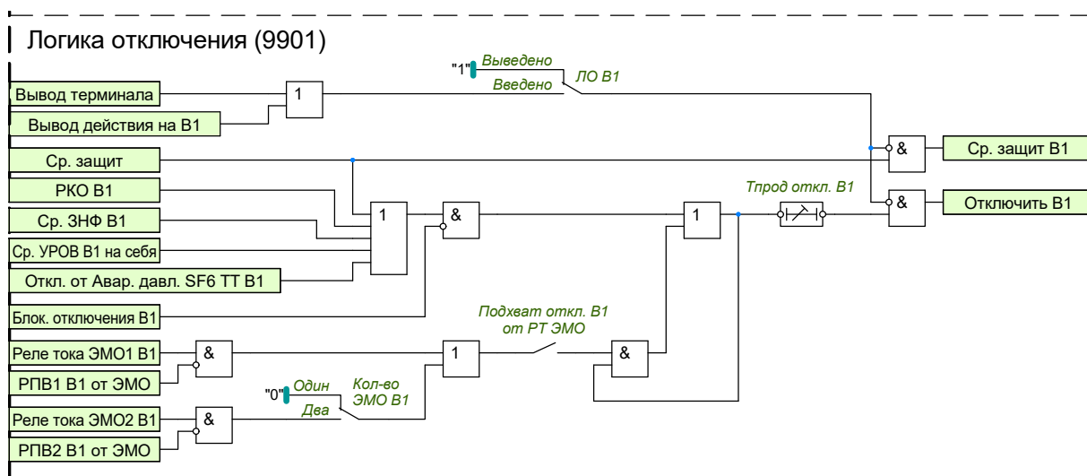
Рисунок 1.51 – Функциональная схема логики отключения В1
