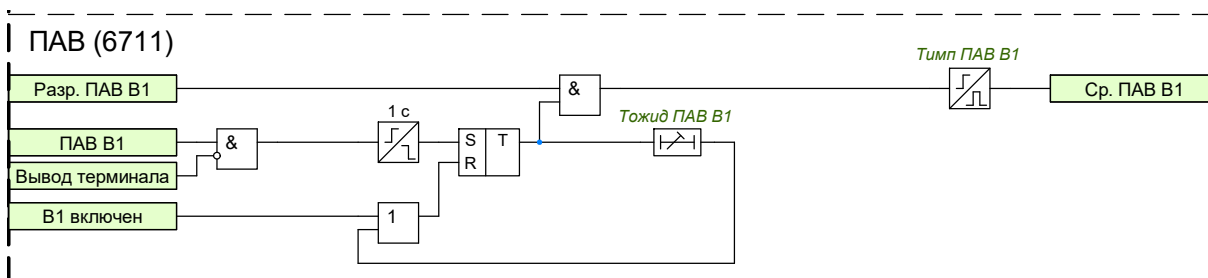
Рисунок 1.44 – Функциональная схема логики ПАВ В1
