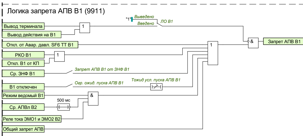
Рисунок 1.43 – Функциональная схема запрета АПВ В1
