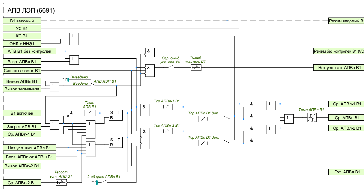
Рисунок 1.40 – Функциональная схема логики АПВ В1 ЛЭП
