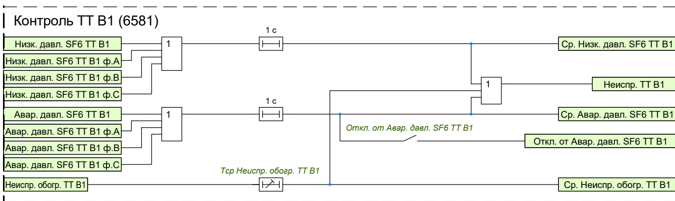
Рисунок 1.46 – Функциональная схема контроля ТТ В1
